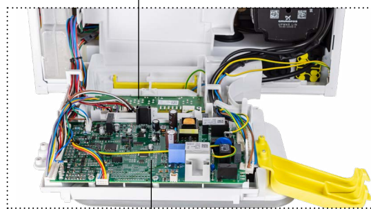
Carte électronique principale
