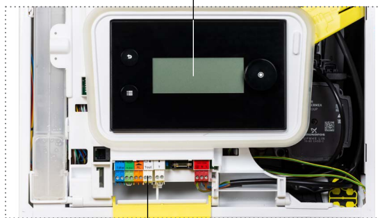
Bornier à vis de raccords électriques
